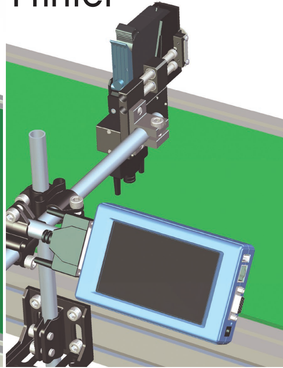
Elfin ID-C Uneven Surface Inkjet Printer
